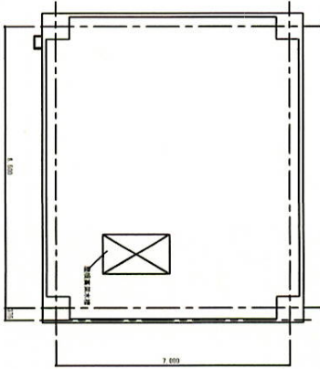
P.H.平面図
