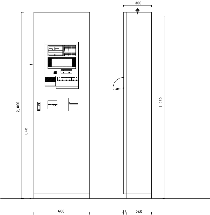
R 型受信機姿図
